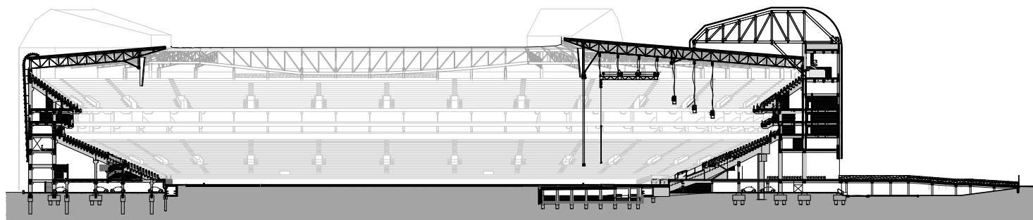
CORTE LONGITUDINAL
