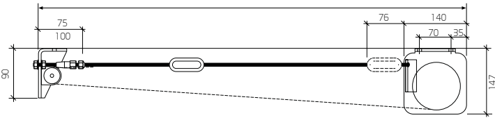
VISTA LATERAL
