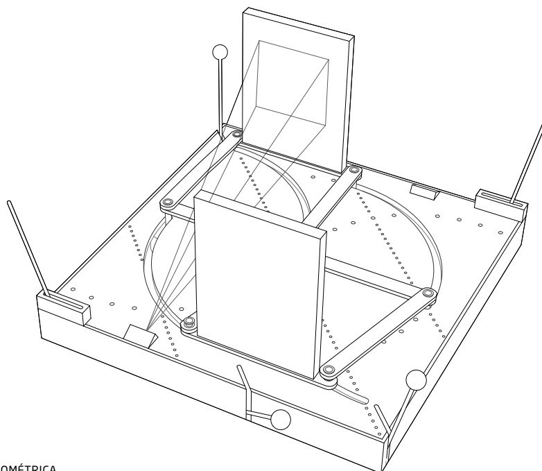
AXONOMÉTRICA
