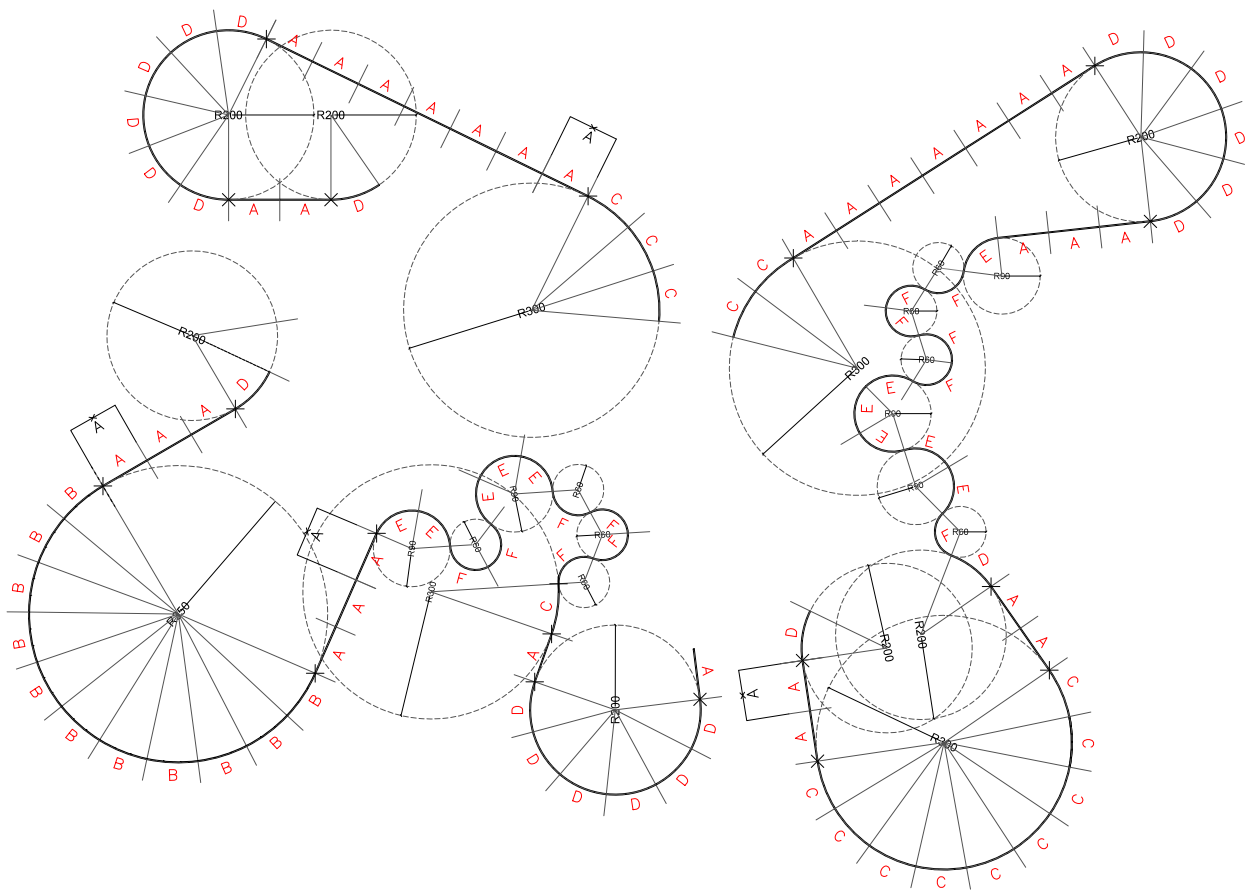
PLANTA TRAZADO
