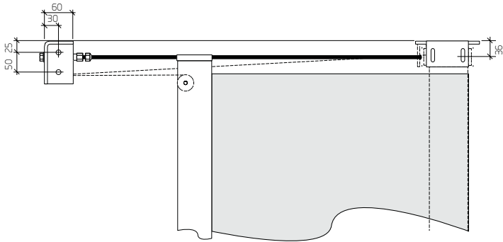
VISTA INFERIOR
