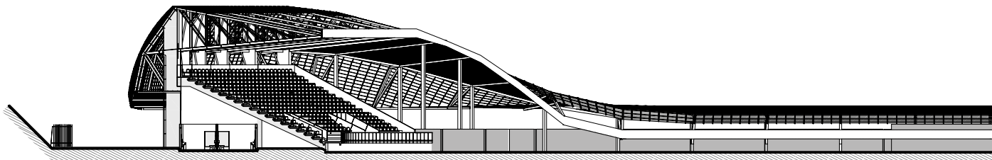
CORTE LONGITUDINAL
