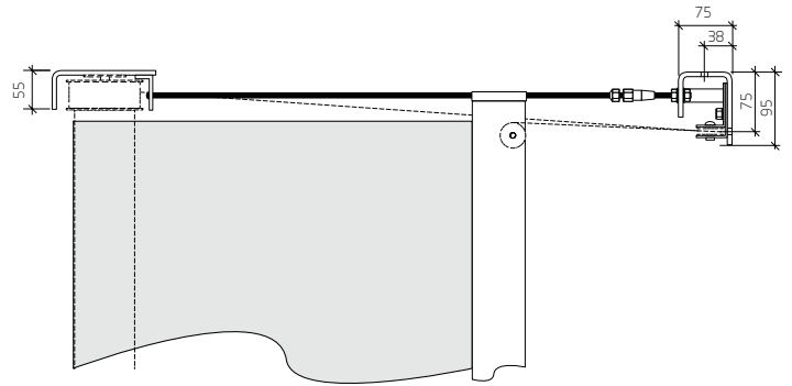
VISTA INFERIOR
