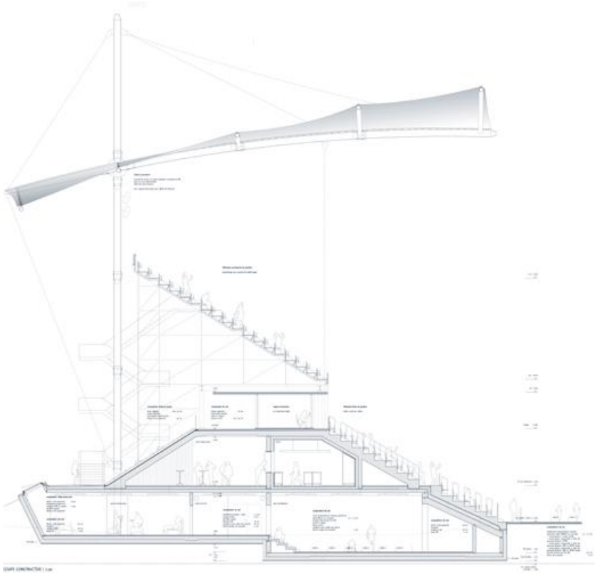
Coupe structurelle
