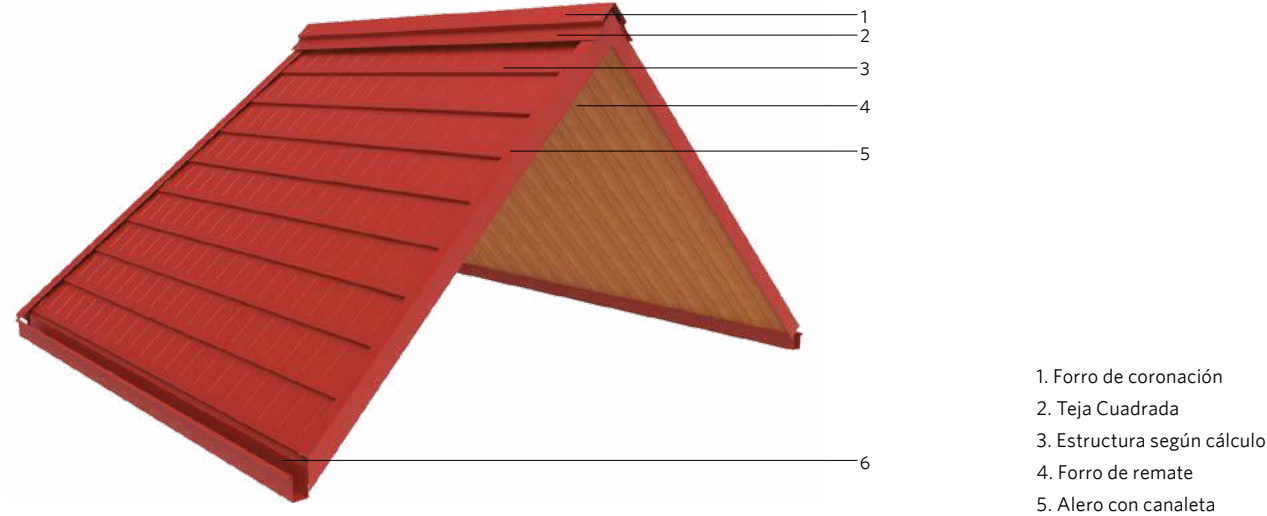
ISOMÉTRICA DE DETALLES
