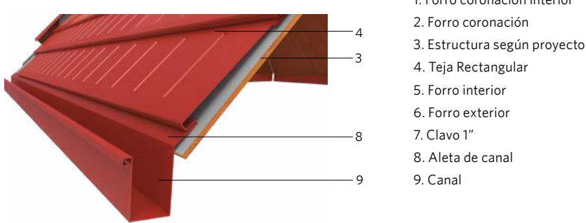
VISTA DETALLE CANALETA
