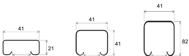
Dimensions PS 21
