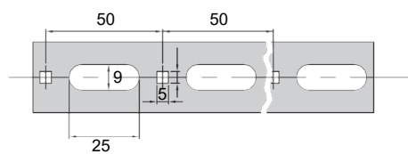
Longueur PS 634
