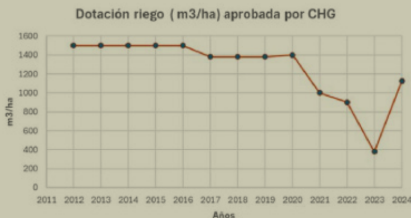
Figura 2: Evolución de la dotación de agua (m³) aprobada por CHG.
