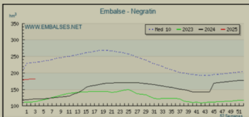
Figura 1: Agua embalsada en la presa del Negratín
