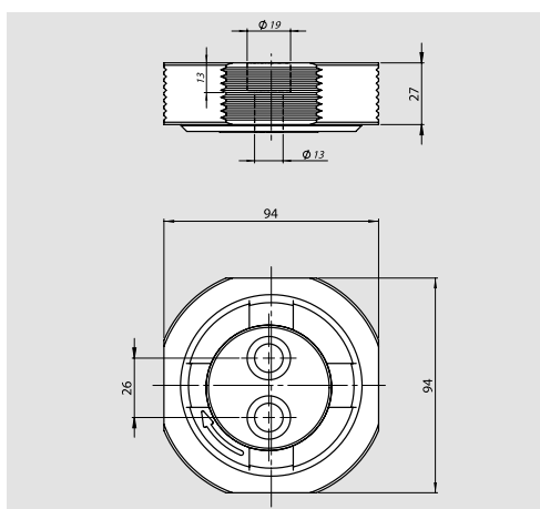
CAM SYSTEM "t" singolo
