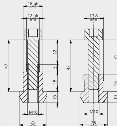
► T-SLOT 18 46204102
