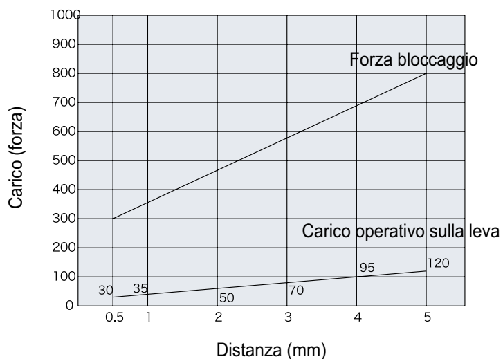
Staffa pivotante tipo 150
