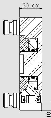
SEZIONE B-B
