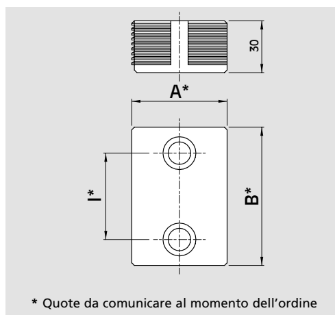
Riscontro CAM SYSTEM "g"
