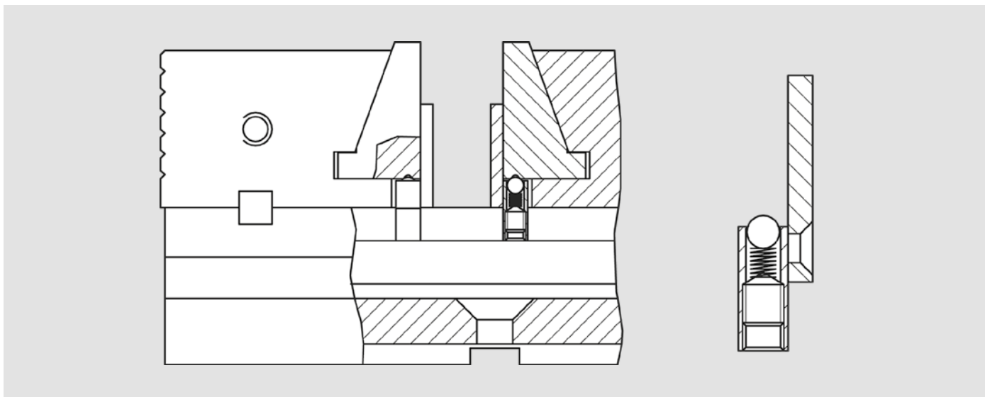
Sistema CLAK SYSTEM per morsa OML
