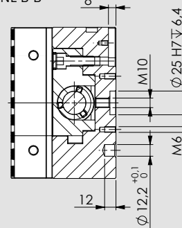
SEZIONE B-B
