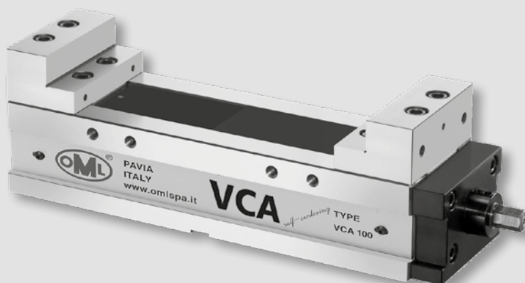
Con ganasce a L
