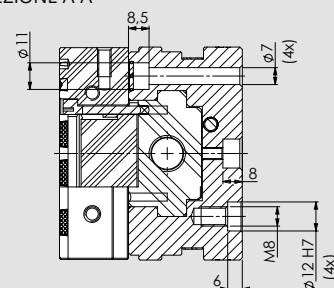
SEZIONE A-A
