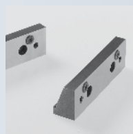
Coppia di ganasce con inserti UGE
