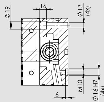
SEZIONE B-B
