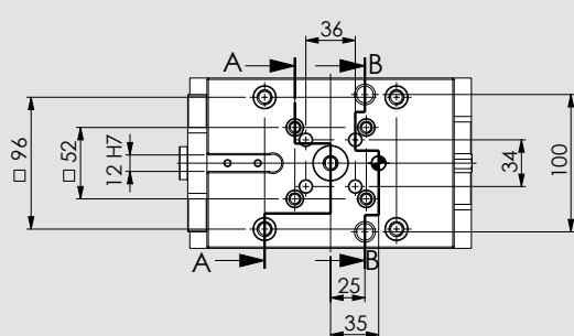
SEZIONE A-A
