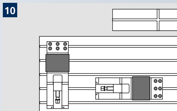
Sedi incrociate per chiavette di posizionamento su tavola m.u.
