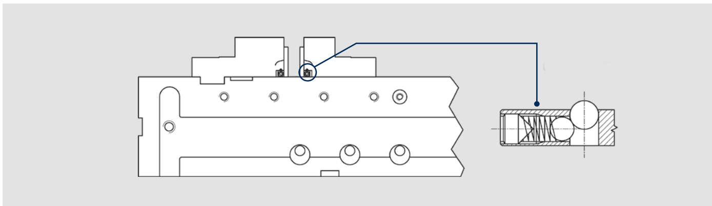
Sistema CLAK SYSTEM universale
