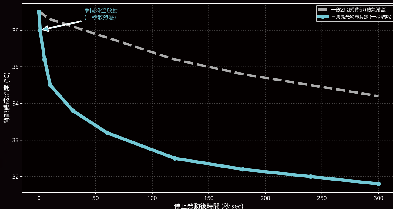
背部透氣設計：散熱效率曲線對比
