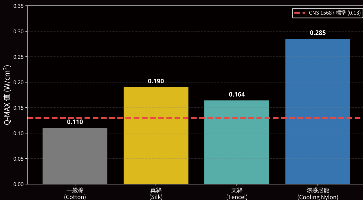
Q-MAX 瞬間涼感值對比圖
