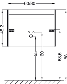
SCHÉMAS TECHNIQUES
