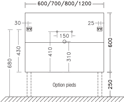
SCHÉMAS TECHNIQUES
